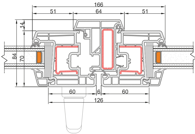
Nodo Centrale Anta squadrata
