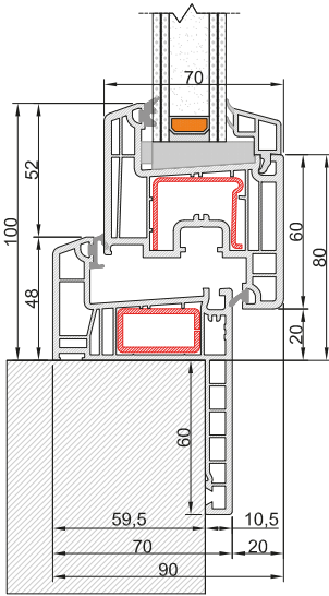
Nodo Inferiore Anta squadrata Telaio Z60
