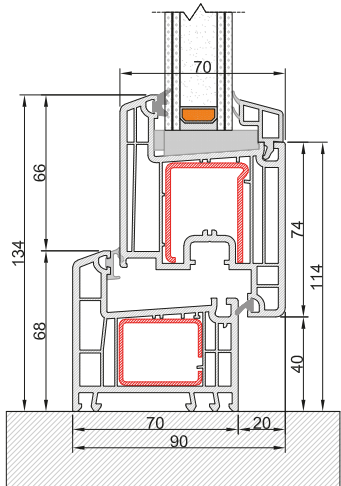
Nodo Inferiore Anta maggiorata Telaio L
