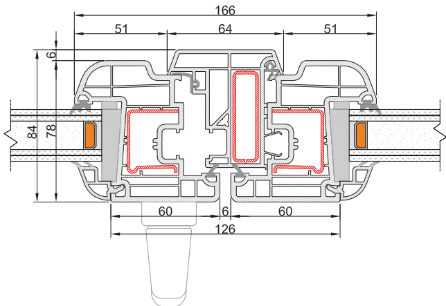
Nodo Centrale Anta arrotondata
