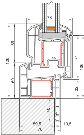
Nodo Inferiore Anta maggiorata Telaio Z40
