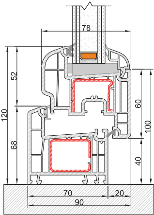
Nodo Inferiore Anta arrotondata Telaio L
