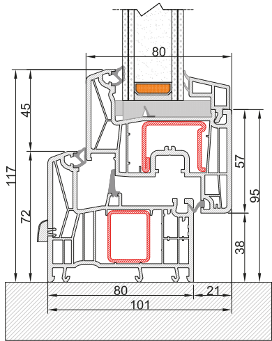
Nodo Inferiore Telaio L
