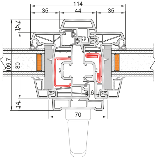
Nodo Centrale Anta slim
