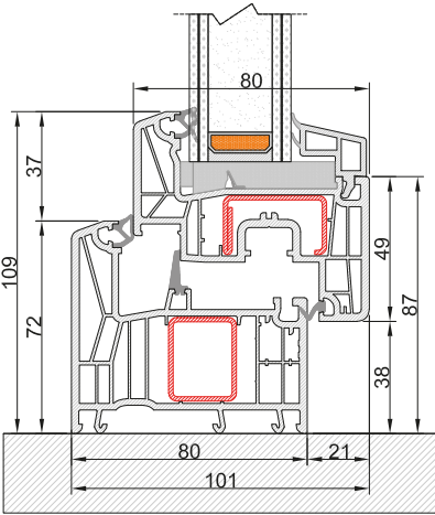
Nodo Inferiore Anta slim
