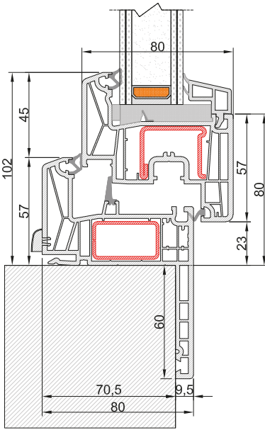
Nodo Centrale Anta slim
