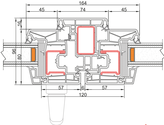
Nodo Centrale Anta squadrata
