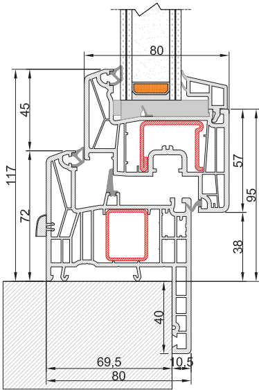
Nodo Inferiore Telaio Z40
